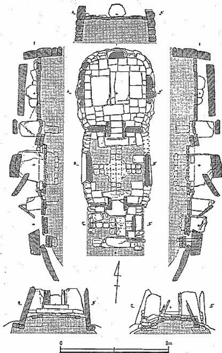
石室平面图
